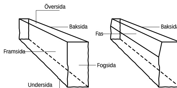
Fig 6.4 Benämning av kantstens olika ytor.
