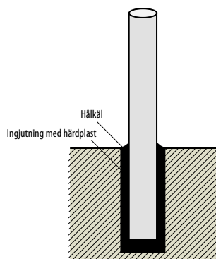
Fig 7.31 Infästning av räcke i sten. Ingjutningen med hårdplast dras upp till ett hålkäl.
