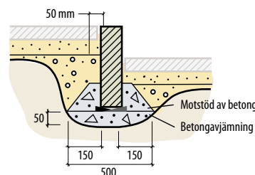
Fig 6.18 Typkonstruktion KB
