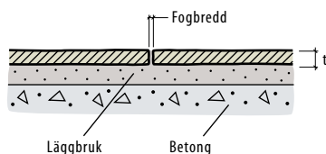
Fig 4.21 Läggnings av hällar i bruk på underlag av betong.
