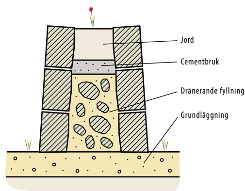
Fig 8.30 Dubbelsidig kallmur av block med plantering i ovasidan.
