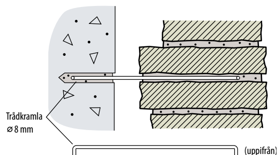
Fig 3.7 Hållarkramla av rundstång, ingjuten i betongstomme, monterad i fogar i mur av skivor (uppiifrån)
