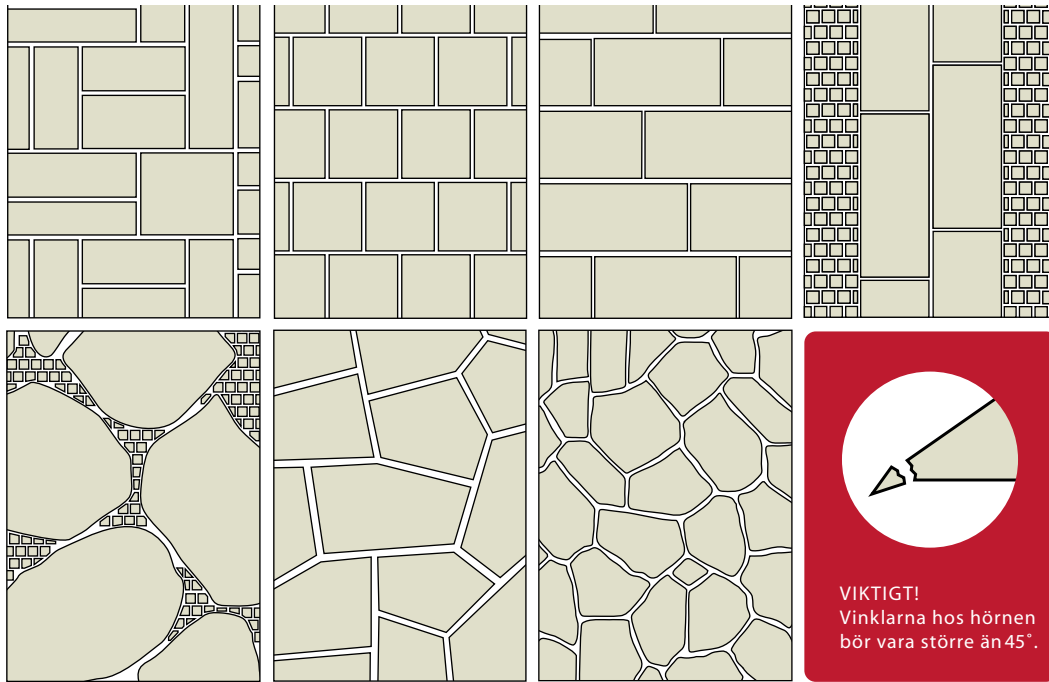
Fig 4.5 Olika läggningssmönster
