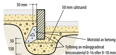
Fig 6.17 Typkonstruktion KG
