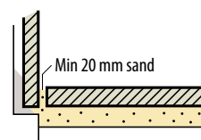
Fig 4.34 Anslutning av beläggning mot byggnad bör utföras med rörelsemån,
