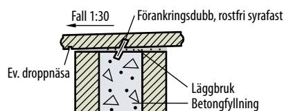
Fig 8.45 Avtäckning på dubbelsidig beklädnadsmur.
