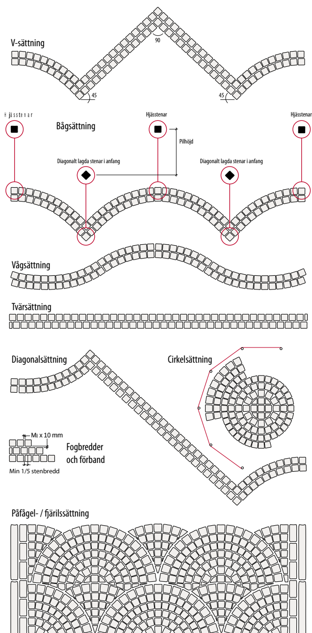
Fig 5.3 Principer för olika mönstersättningar med gatsten.
